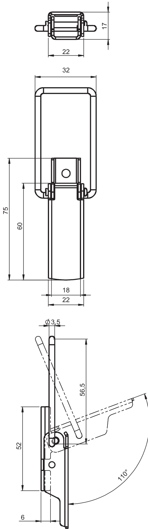
7404 - Latch
