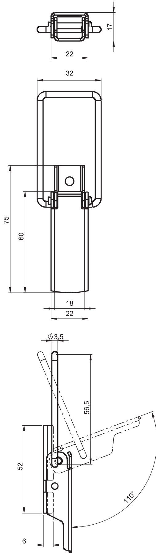
7404 - Latch
