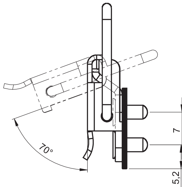
7407 - Latch
