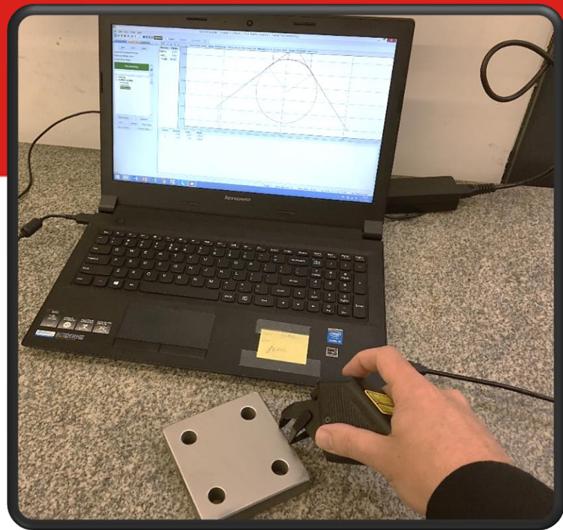
Dispozitivul HS722 de masurare cu laser
